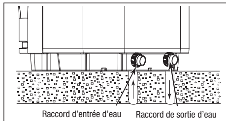
Figure 14. Hiverner la thermopompe JRT
