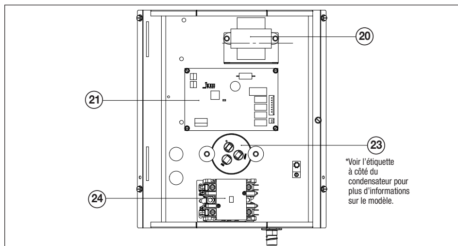
Figure 16. Boîte électrique monophasée pour Jandy JRT
