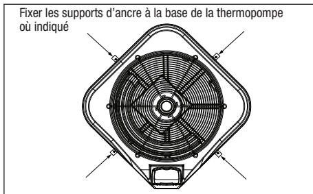
Figure 2. Positions de la bride d'ancrage
