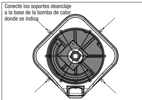
Figura 2. Posiciones de las abrazaderas de anclaje
