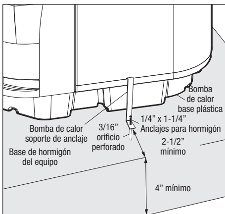
Figura 3. Instalación de las abrazaderas de anclaje
