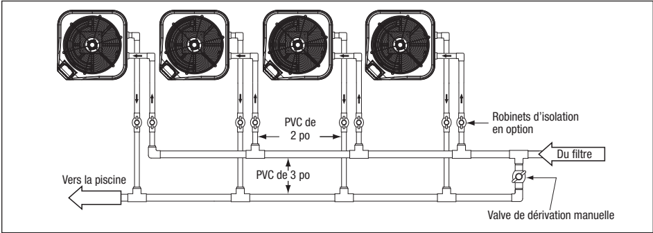
Figure 7. Disposition de la plomberie de quatre (4) thermopompes
