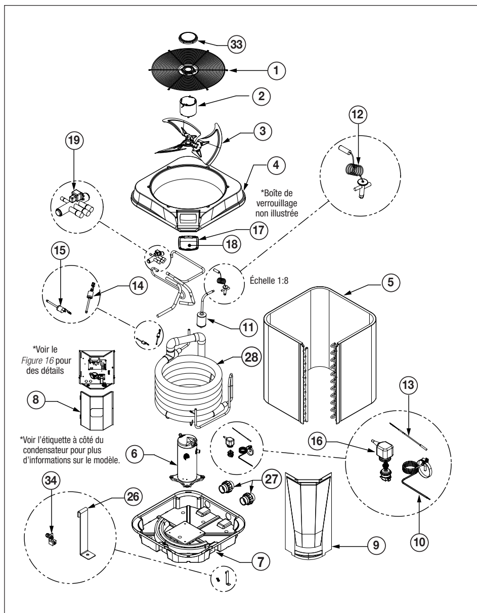
Figure 15. Vue agrandie des thermopompes Jandy JRT (JRT2000R illustrée)
