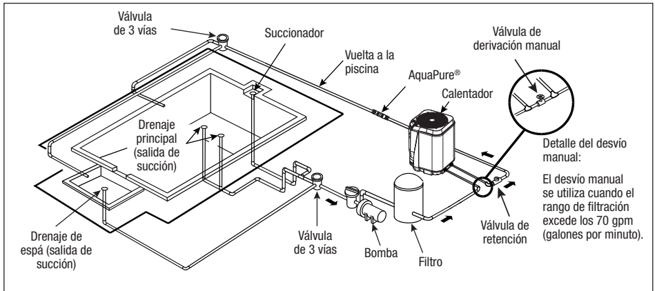
Figura 4. Disposición estándar de las tuberías
