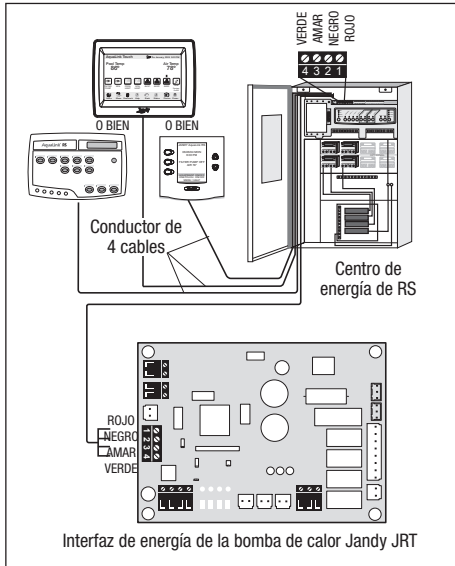
Figura 12. Bomba de calor Jandy JRT a centro de energía, conexión RS485 (4 cables)
