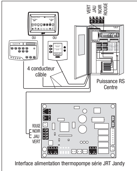
Figure 12. Thermopompe Jandy JRT à centre d'alimentation - connexion RS485 (4 fils)
