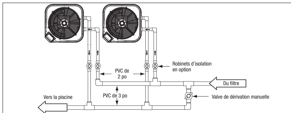
Figure 6. Disposition de la plomberie de deux (2) thermopompes
