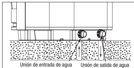
Figura 14. Preparación de la bomba de calor JRT para el invierno
