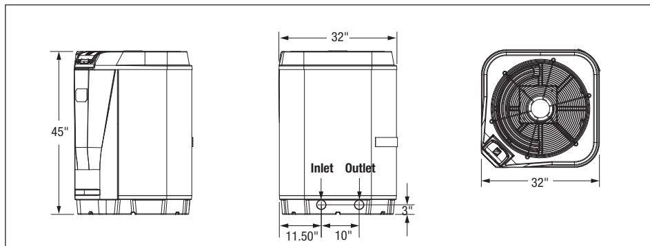
Figure 1. Dimensions des thermopompes JRT de Jandy
