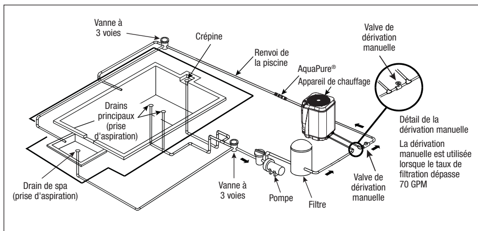
Figure 4. Disposition normale de la plomberie
