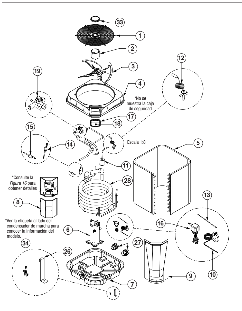
Figura 15. Bombas de calor Jandy JRT, vista ampliada (se muestra la JRT2000R)
