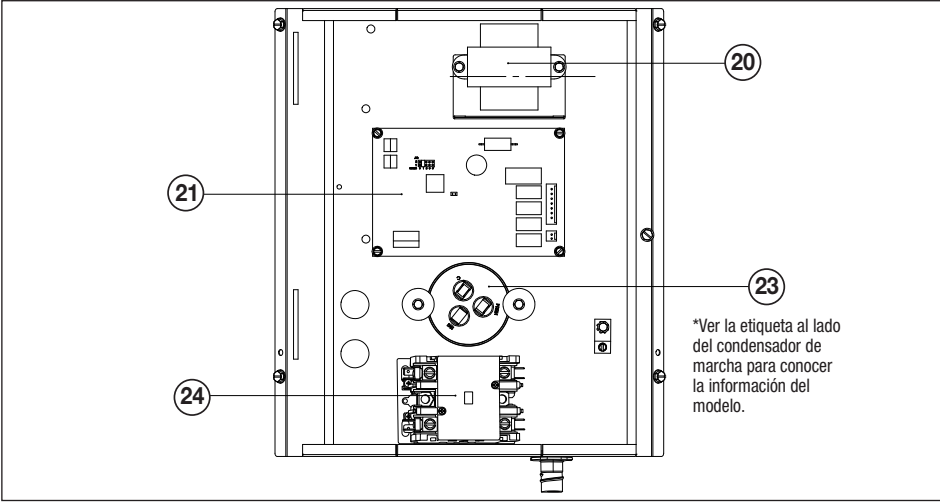
Figura 16. Caja de electricidad monofásica de Jandy JRT
