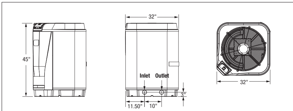
Figura 1. Dimensiones de las bombas de calor Jandy JRT
